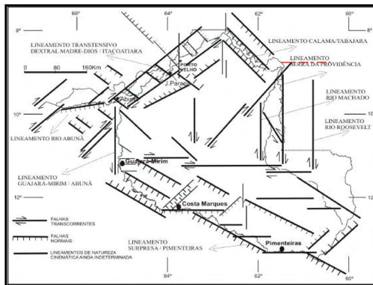
FIGURA B.III. 9 – Quadro geral da neotectônica no estado de Rondônia e adjacências
