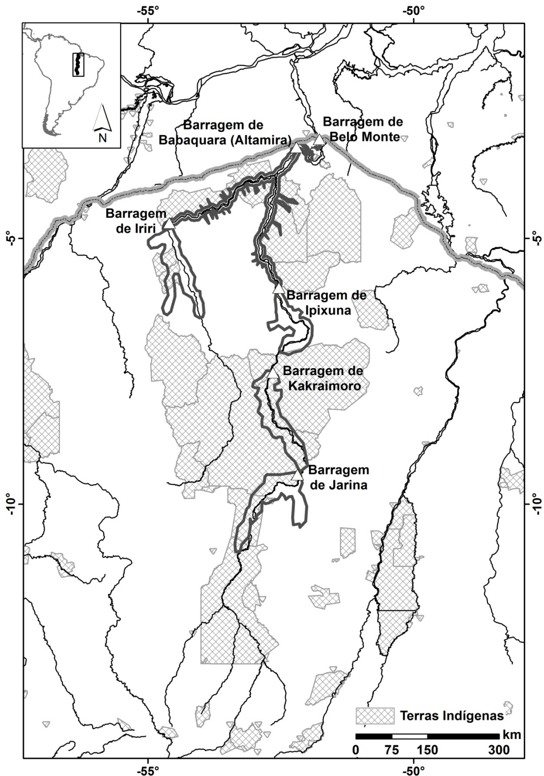
Figura 1 – Barragens e contornos dos reservatórios originalmente planejados para a bacia do Rio Xingu. Áreas indígenas estão hachura cruzada. A questão de se barragens rio acima de Belo Monte serão posteriormente construídas, que as autoridades do governo brasileiro atualmente negam, é uma parte crítica do debate.
